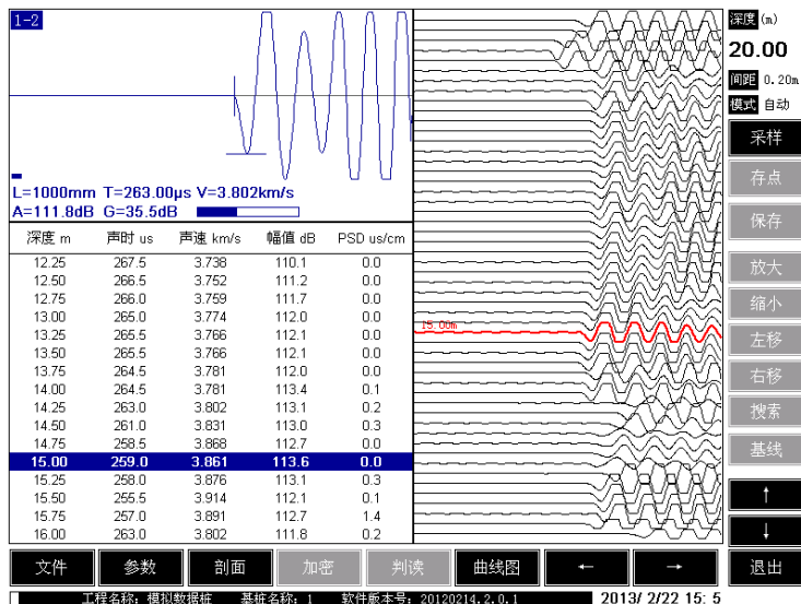
图 5.1-1 测试主界面
