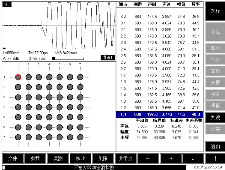
图 7.1-1 测缺主界面
