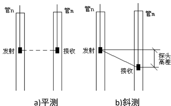
图 5.7-3 测点布置示意图
